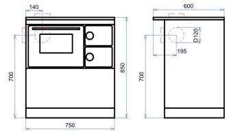
THORMA OKONOM 75 FIKO De Luxe - Levý
